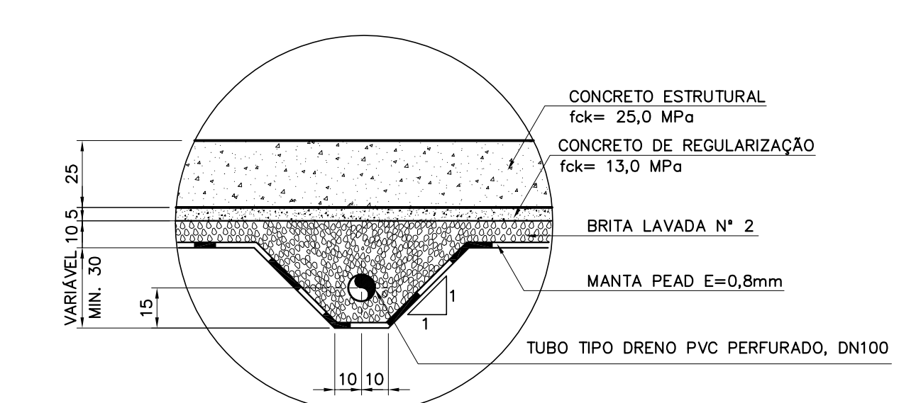
DETALHE 02 DRENO SUBSUPERFICIAL ESC. 1:20
