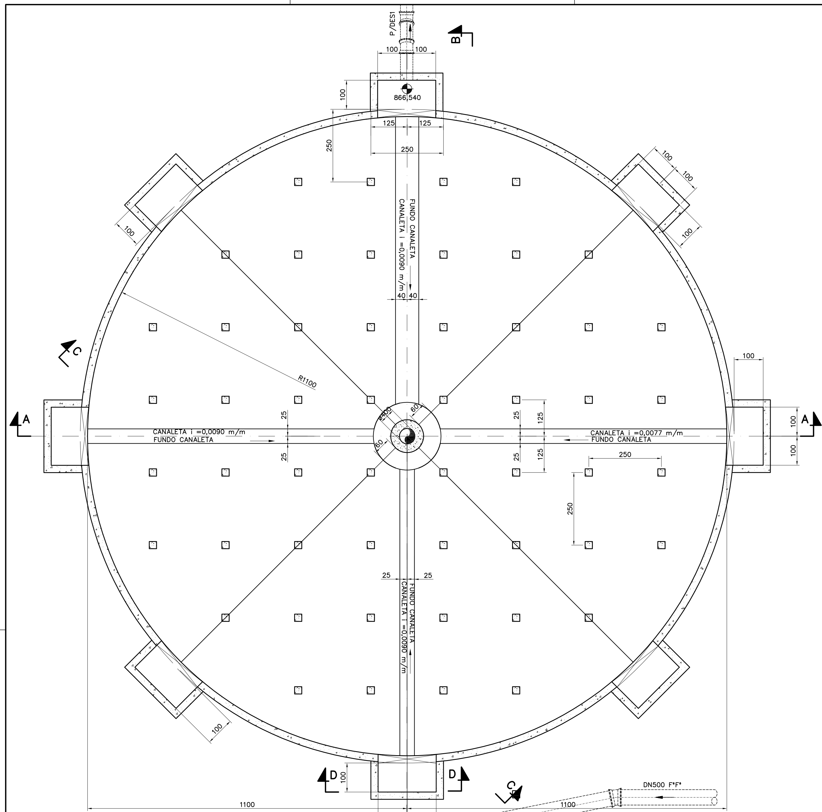
PLANTA NÍVEL INFERIOR ESC. 1:75
