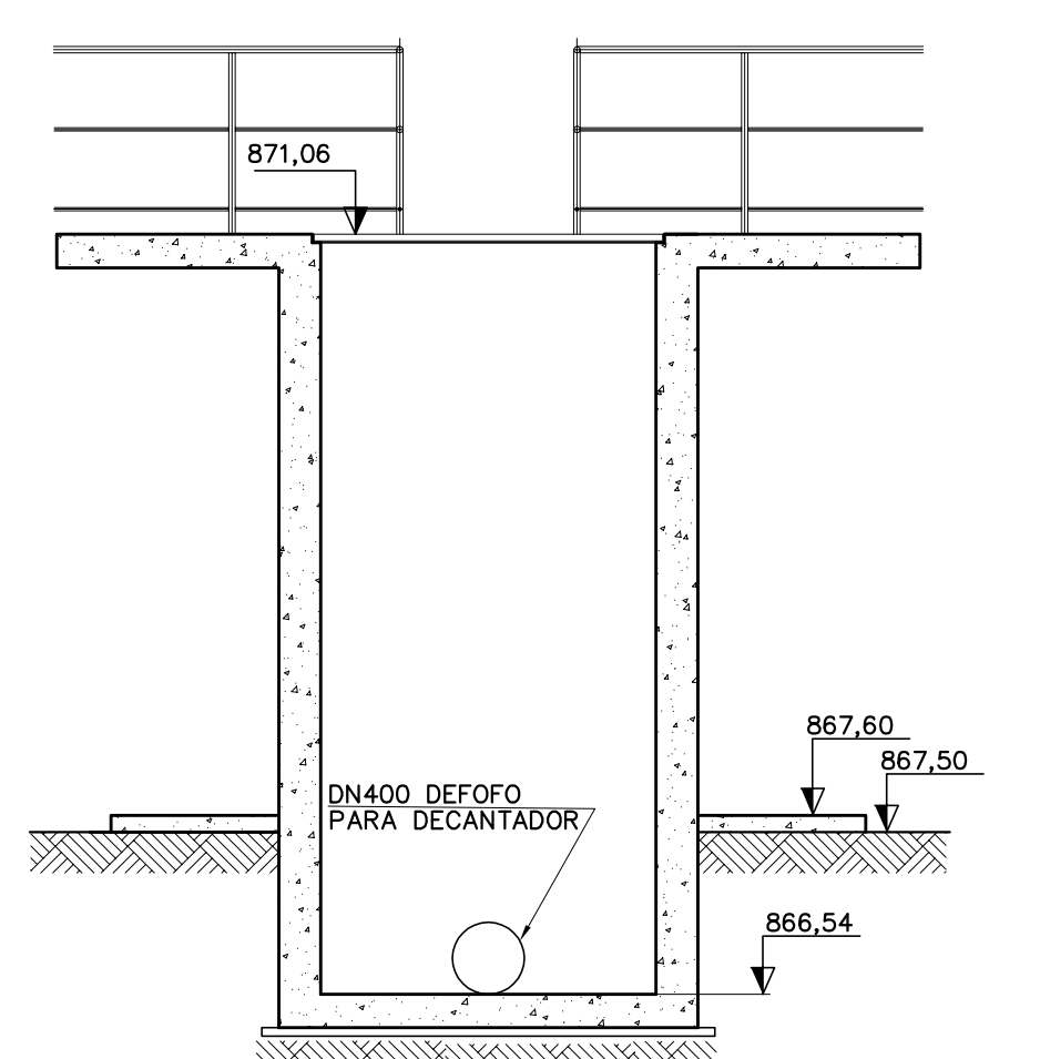
CORTE D-D ESC. 1:50
