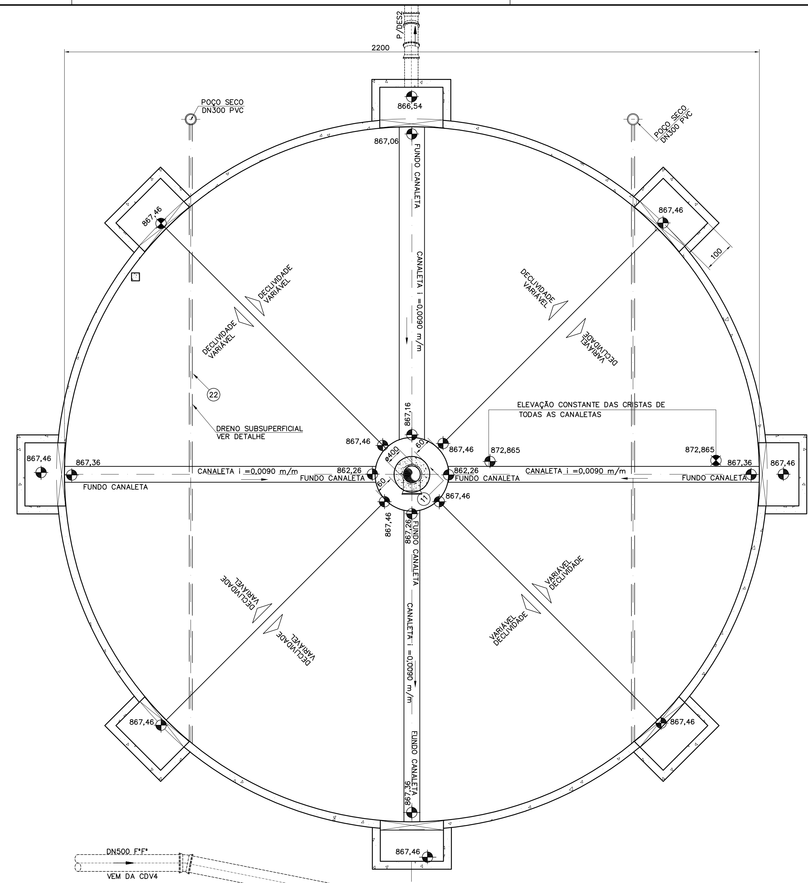
PLANTA DE FUNDO ESC. 1:75
