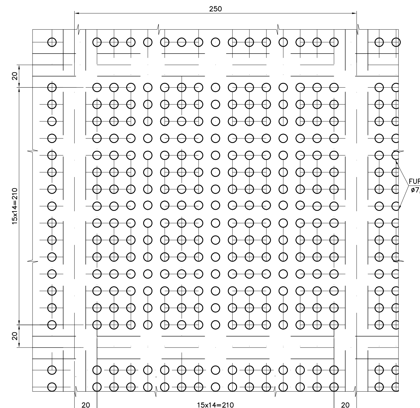
DETALHE 03 LAJE PERFORADA ESC. 1:20
